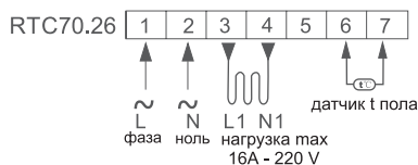
Диаграмма соединения
