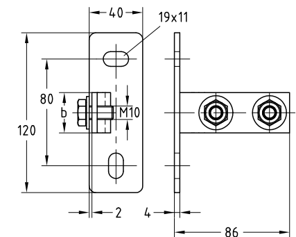
МРС-Торцовый фланец, продольное исполнение
