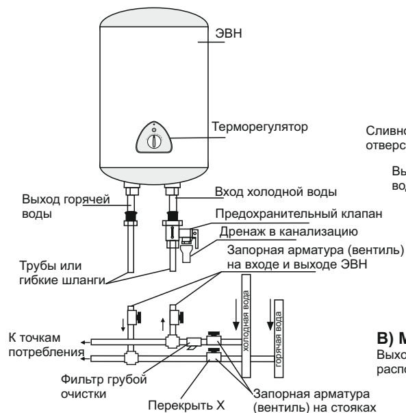
Рис. 2. Схема подключения ЭВН к водопроводу
