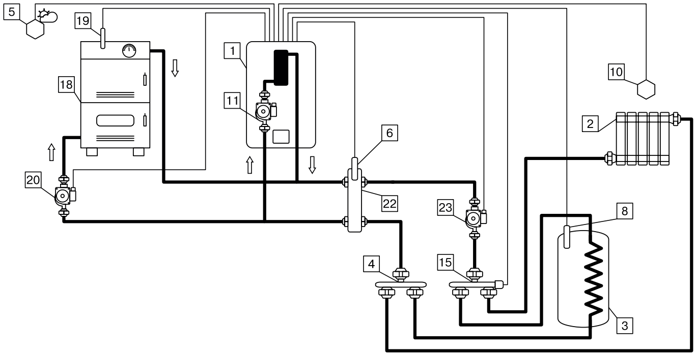
Схема 3 Контур отопления 2 и контур трехходового смесительного клапана в режиме теплого пола
