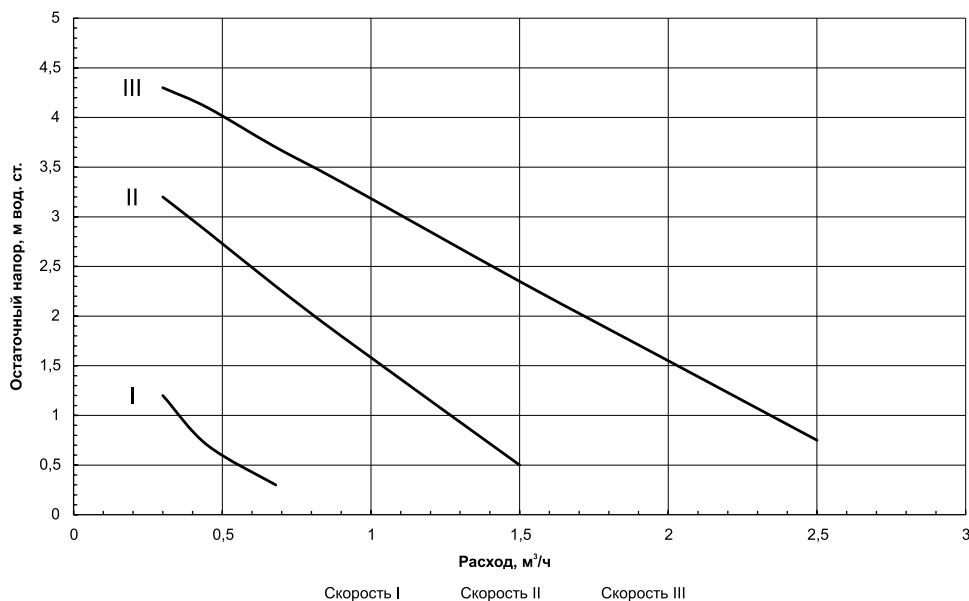
Рис.1 Остаточный напор для циркуляционного насоса ZOTA Ring 25/60 (Для котлов MK-S Plus 6-21)
