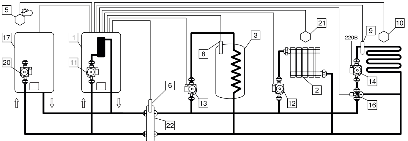
Схема 3.1 Контур отопления 2 и контур трехходового смесительного клапана в режиме отопления
