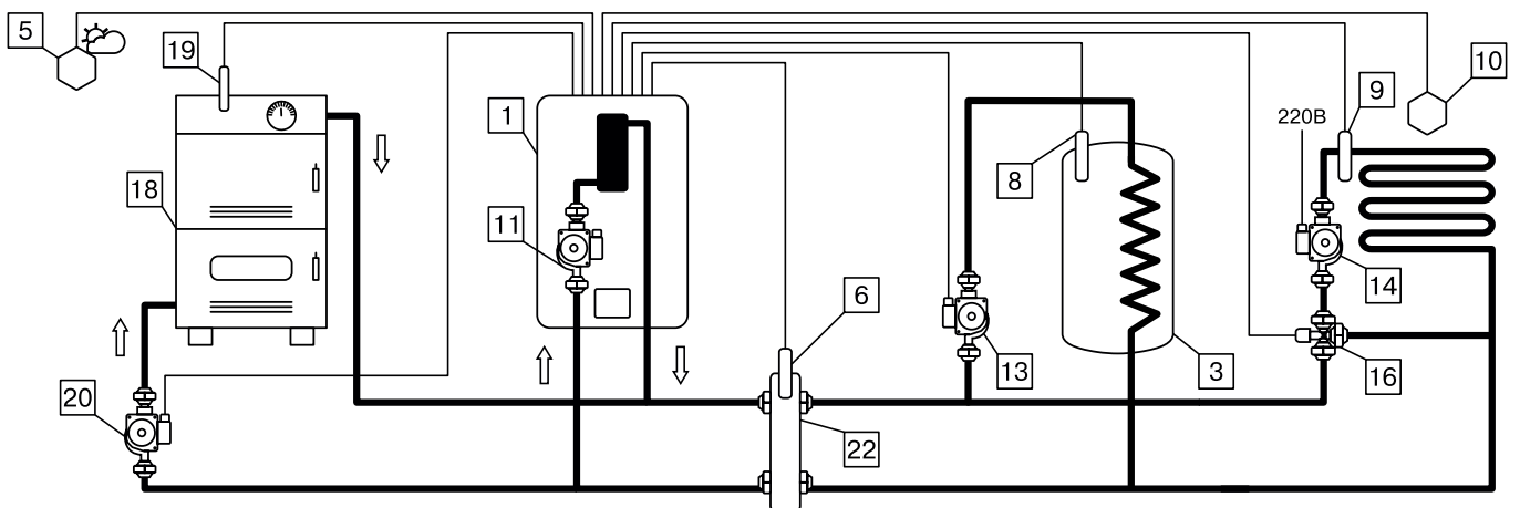
Схема 3.2 Контур ГВС и контур трехходового смесительного клапана в режиме отопления
