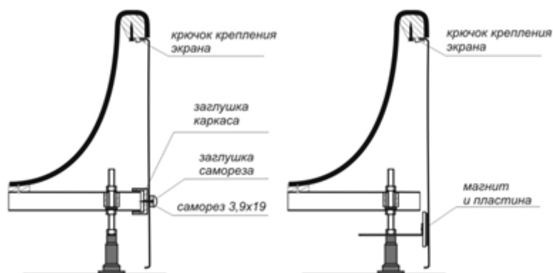
Установка декоративной панели Рис. 1.
