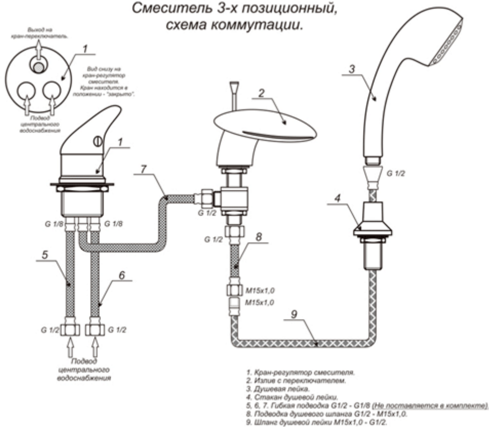
Схема подключения 3-х позиционного смесителя Рис. 3.1
