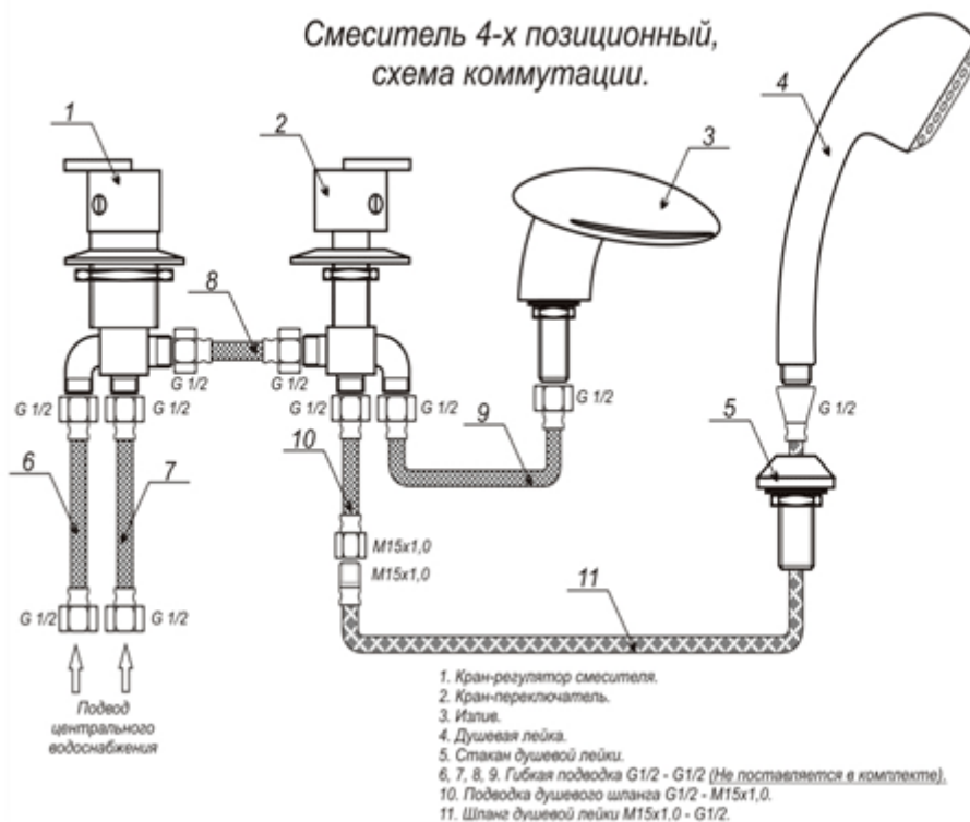
Схема подключения 4-х позиционного смесителя Рис. 3.2
