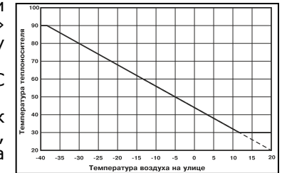
График погодозависимого регулирования.
