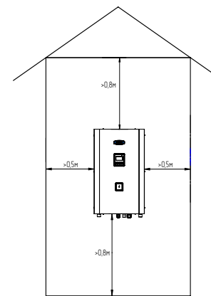
Рис.4 Схема установки миникотельной
