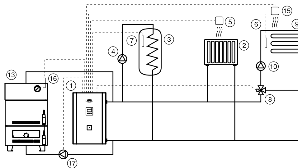
Рис.6 Упрощенная схема подключения миникотельной в режиме вспомогательного с контуром ГВС и тёплого пола
