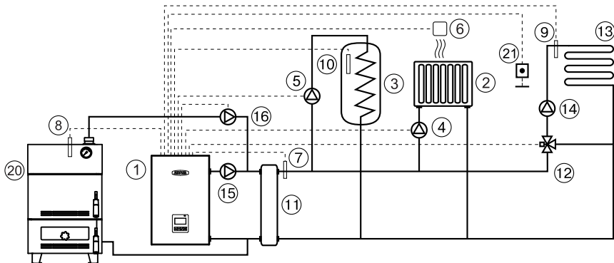
Рис.11 Упрощенная схема подключения котла в режиме вспомогательного с гидроразделителем, контуром ГВС, контуром отопления и тёплого пола.
