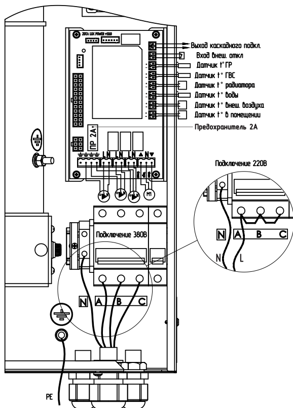
Рис. 3 Схема подключения электроводонагревателя
