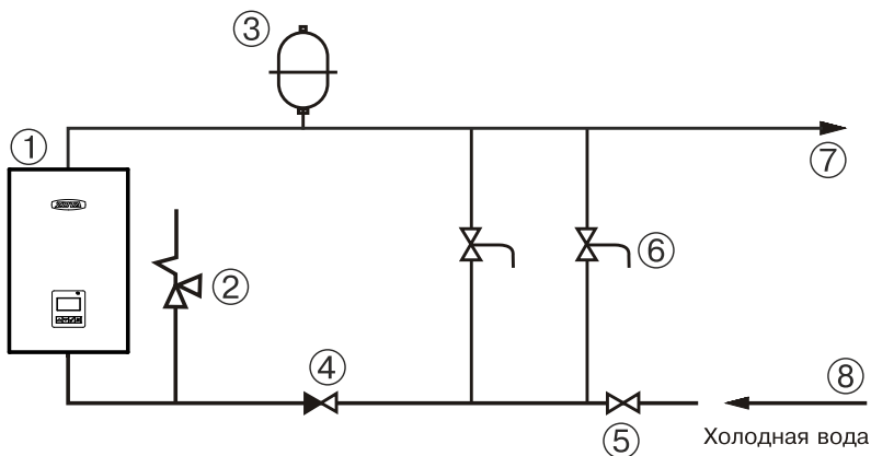
Рис. 12 Упрощенная схема подключения в качестве электроводонагревателя с проточным режимом работы
