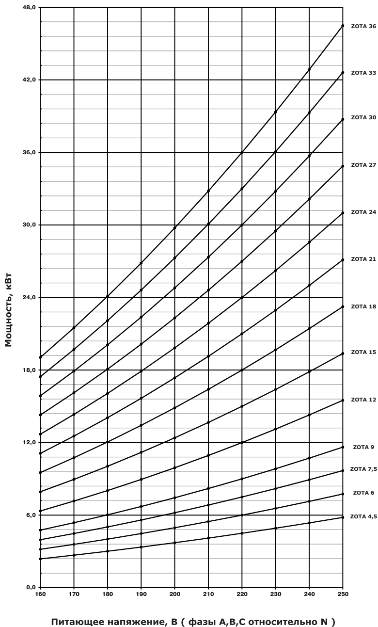
Рис. 13 График изменения мощности электроводонагревателя в зависимости от питающего напряжения
