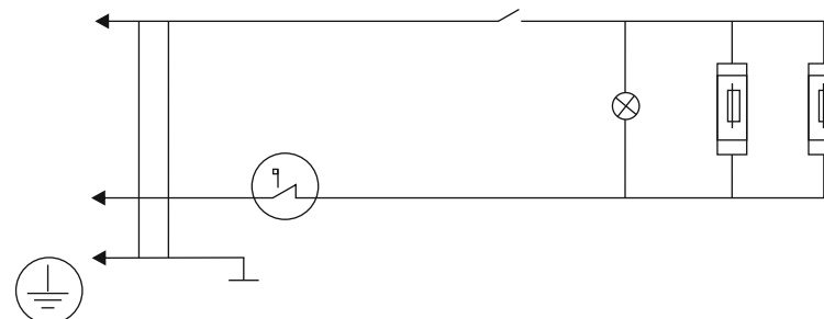
Рис. 2 Схема настенного монтажа электроконвектора
