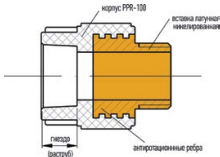
Рис. 2. Комбинированный фитинг в разрезе
