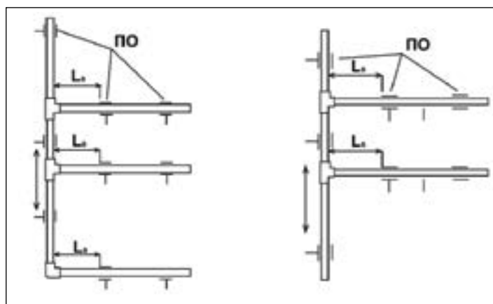
Рис. 14. Пример компенсации стояков у основания и на вершине
