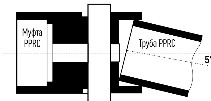
Рис. 22. Отклонение осевой линии трубы от осевой линии нагревательного устройства
