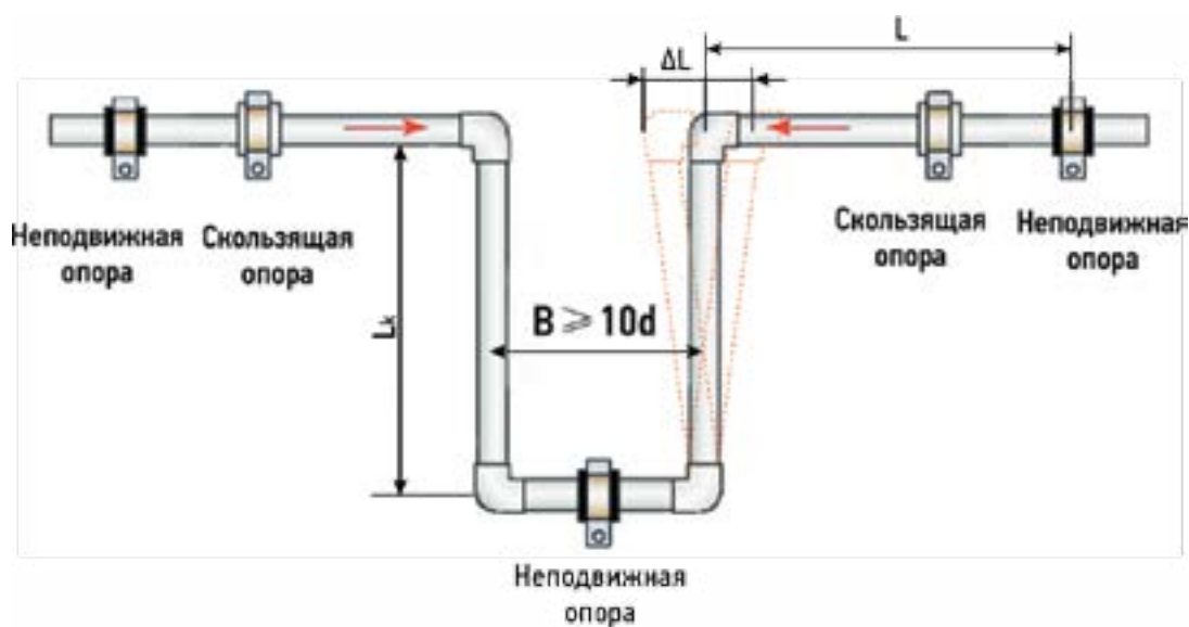
Рис. 9 П-образный элемент трубопровода
