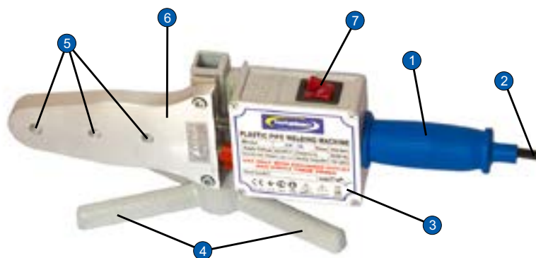
Рис. 17. Устройство сварочного аппарата
