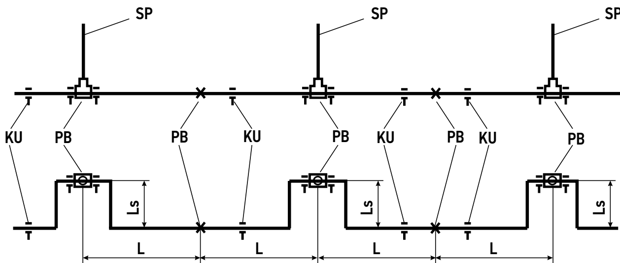
Рис. 13. Компенсация горизонтального трубопровода способом «FV-plast»
