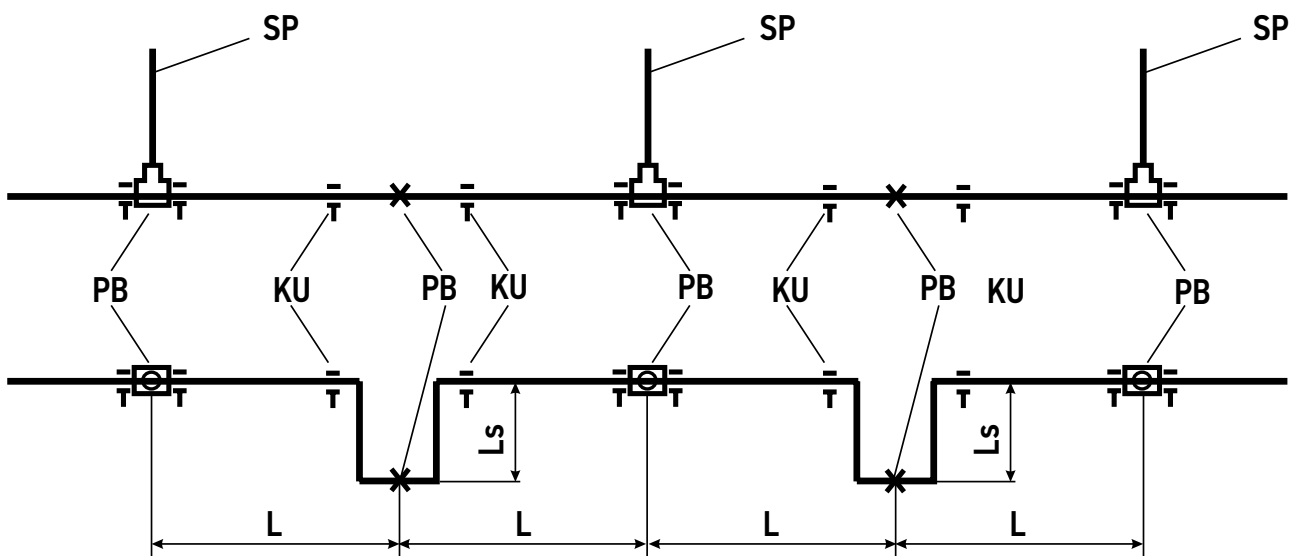
Рис. 13. Классический способ компенсации горизонтального трубопровода
