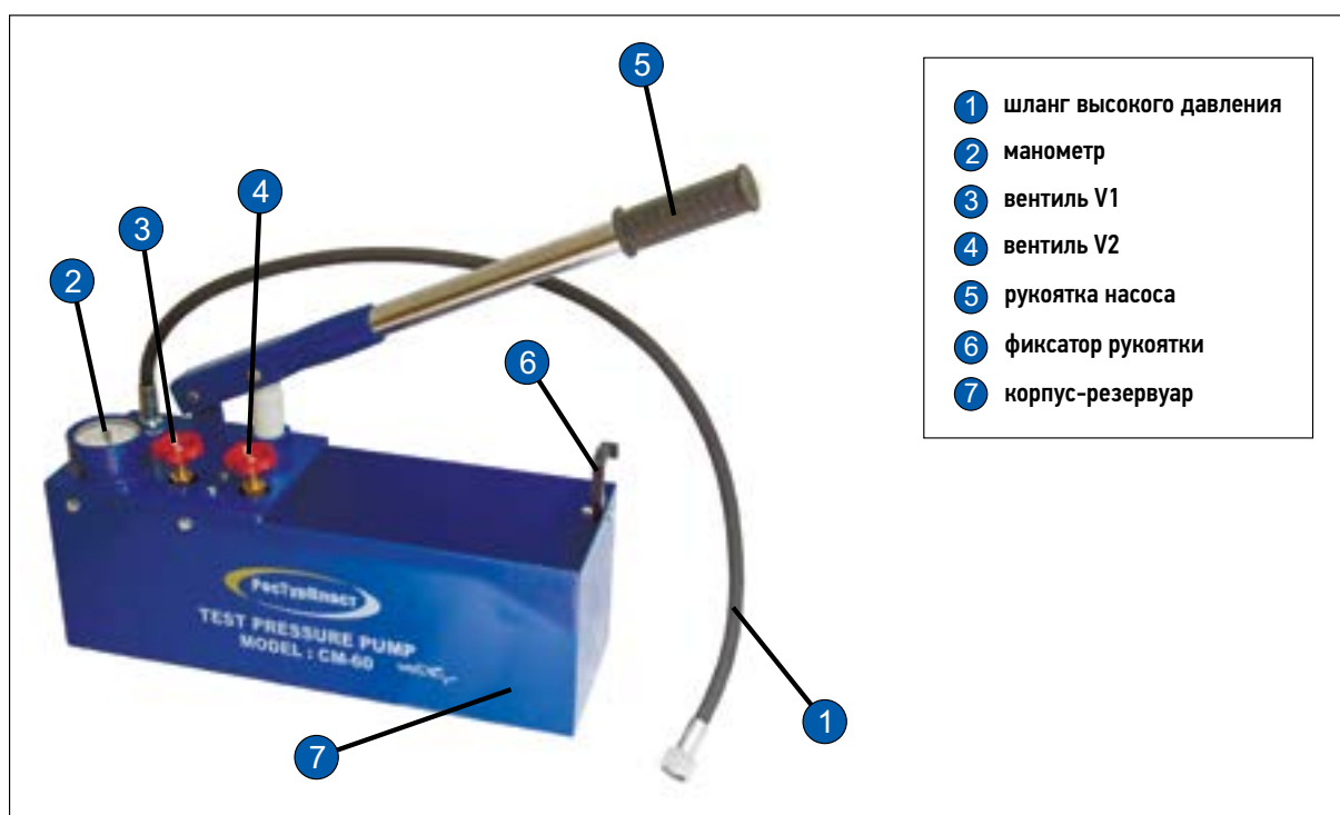
Рис. 19. Оборудование для опрессовки трубопровода (ручной опрессовочный насос).
