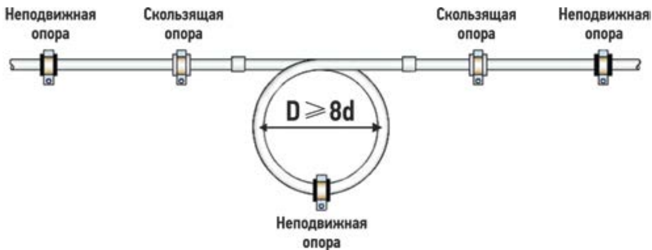
Рис. 11. Петлеобразный компенсатор
