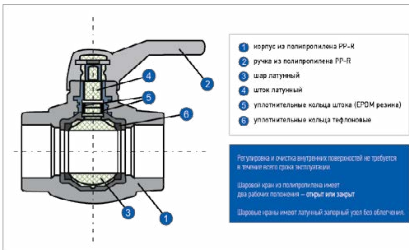
Рис.4. Конструкция шарового крана «Ростурпласт»
