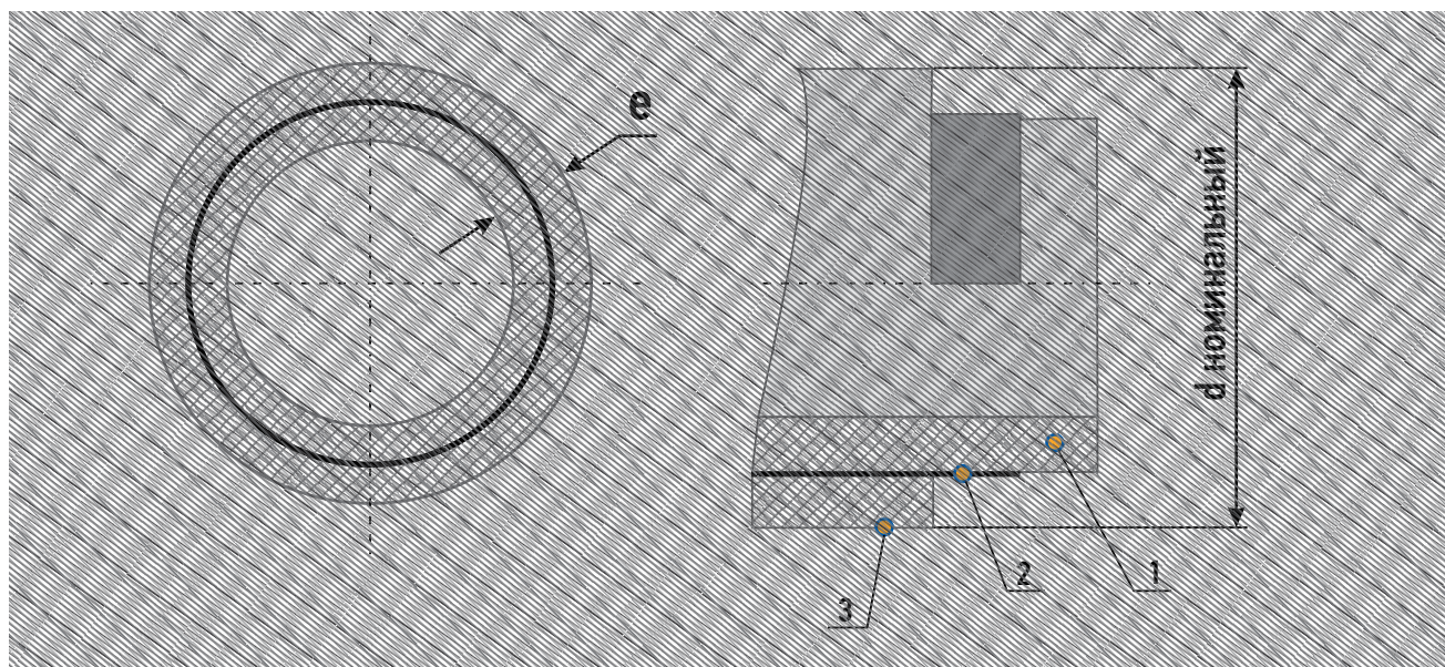
Рис. 1. Схема трубы типа армирования внутри стенки трубы 1 — внутренний слой трубы (PP-R); 2 — алюминиевая фольга (Al); 3 — наружный слой трубы (PP-R); ( e — общая толщина стенки трубы; d_{\text{номинальный}} — номинальный наружный диаметр трубы)
