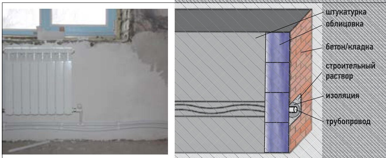
Рис. 16. Пример некомпенсированного трубопровода.
