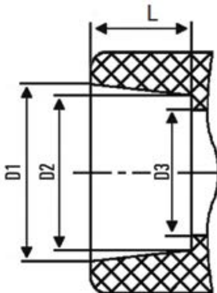
Рис. 3. Раструбная часть фитингов
