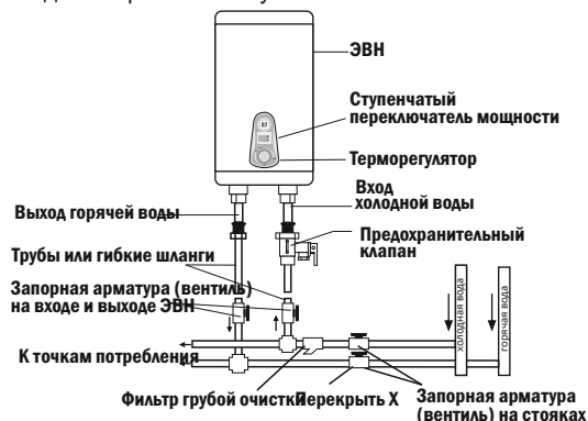
Рис. 2. Схема подключения ЭВН к водопроводу
