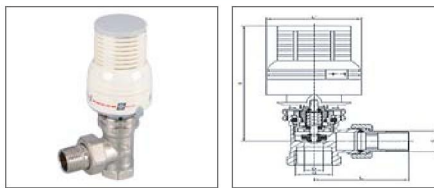
КЛАПАН УГЛОВОЙ С ТЕРМОГОЛОВКОЙ AxTSP
