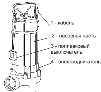
Рис. 2 Устройство насоса
