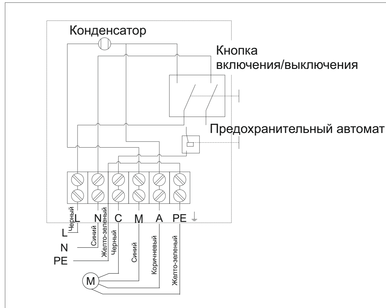
Схема подключения ПЗУ
