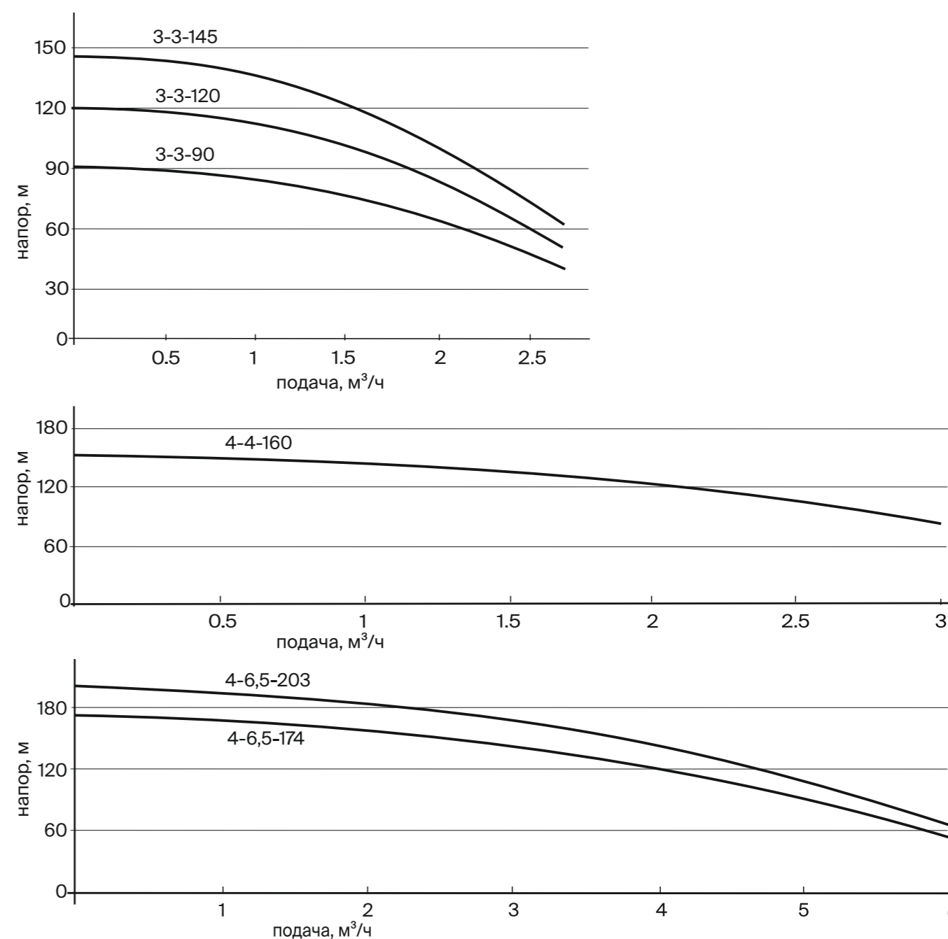
Рисунок 1. Напорно-расходные характеристики насоса
