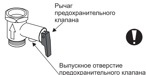
Рис. 3. Предохранительный клапан
