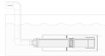
Рисунок 9. Монтаж насоса в охлаждающем кожухе
